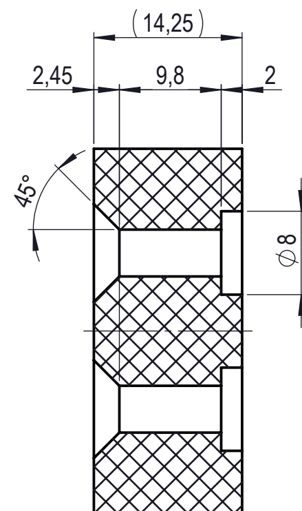
COUPE A-A
